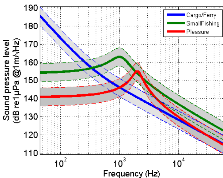
Figure 21 : Gabarit et tirages des spectres de niveaux de bruit émis par les navires (en dB réf. 1μPa/VHz @1m) en fonction de la fréquence et de leur catégorie (« Cargo », « Ferry », « Pêche », « Plaisance »). Les barres d'erreurs (gris) indiquent la variabilité observée dans les tirages aléatoires effectués dans le cadre des scénarios technico-opérationnels. Source Quiet-Oceans d'après (Wales & Heitmeyer, 2002), (Hildebrand, 2009).
